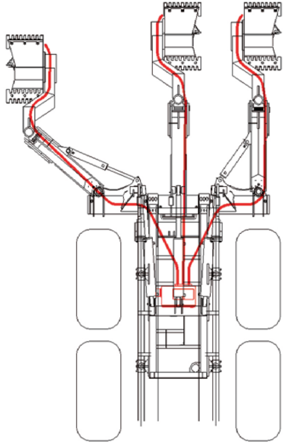
S35.a asennetaan maanmuokkauslaitteeseen, ja siemenet siirretään letkuja pitkin kylvökohteisiin. Kylvöpyörät annostelevat siemenet jokaiseen kylvökanavaan yksitellen.
